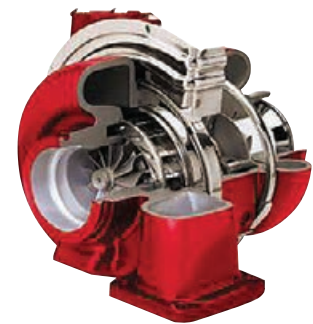
고성능 가변 제어 터보시스템(VGT) 저 RPM에서도 강력한 순간파워와 빠른 작업 응답성 발휘
