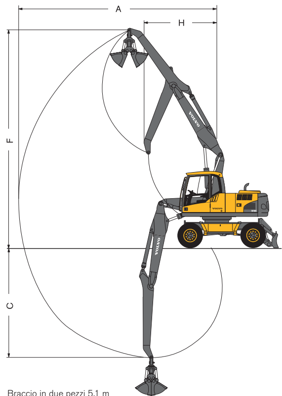
Braccio in due pezzi 5,1 m e avambraccio industriali 2,95 m
