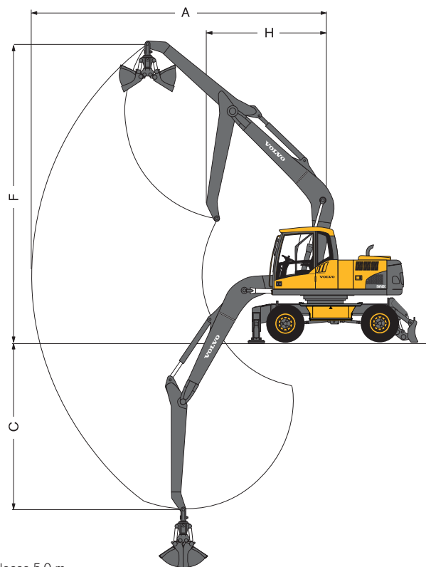
Braccio monoblocco 5,0 m e avambraccio industriali 2,95 m
