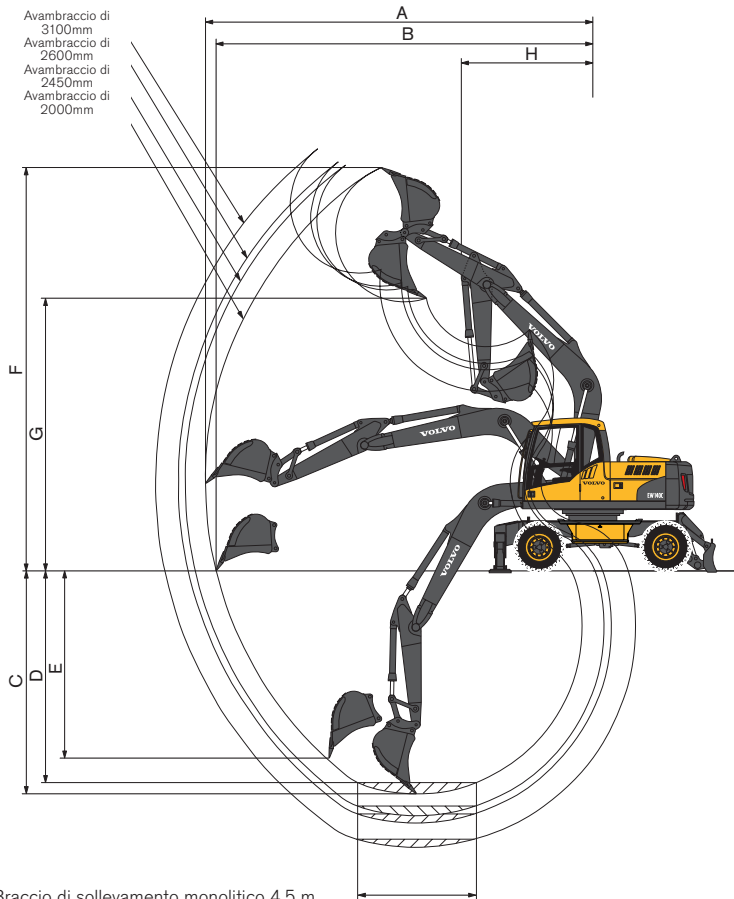
Braccio di sollevamento monolitico 4,5 m e avambraccio 2,0 m, 2,45 m, 2,6 m, 3,1 m
