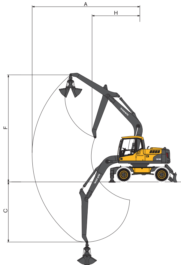
Braccio di sollevamento monolitico 4,5 m e avambraccio industriale 2,95 m
