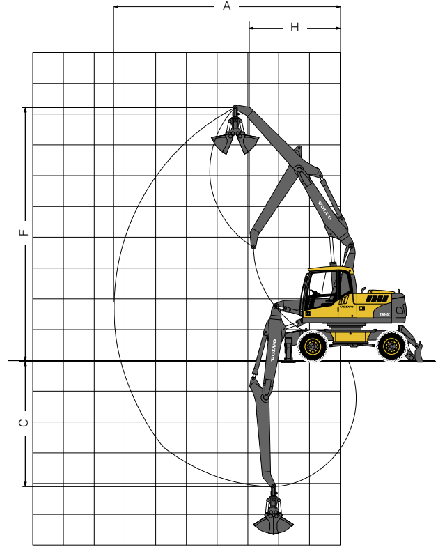
Kaksiosainen puomi 4,7 m ja kahmarin varsi 2,95 m
