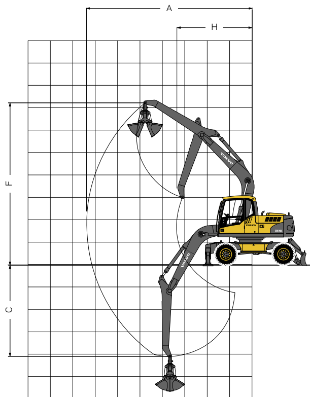
Yksiosainen puomi 4,5 m ja kahmarin varsi 2,95 m
