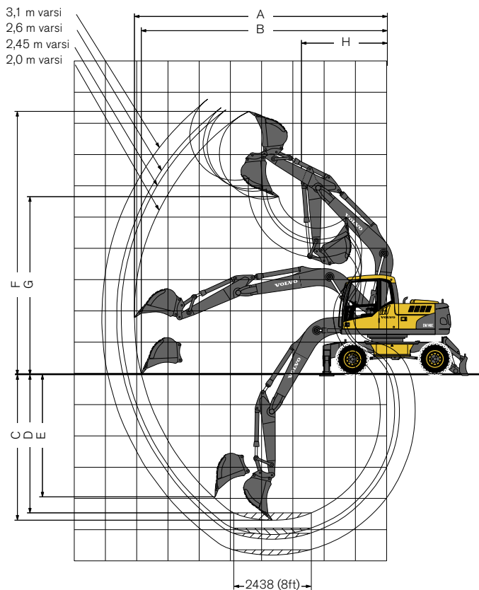
Yksiosainen puomi 4,5 m ja varsi 2,0 m, 2,45 m, 2,6 m ja 3,1 m
