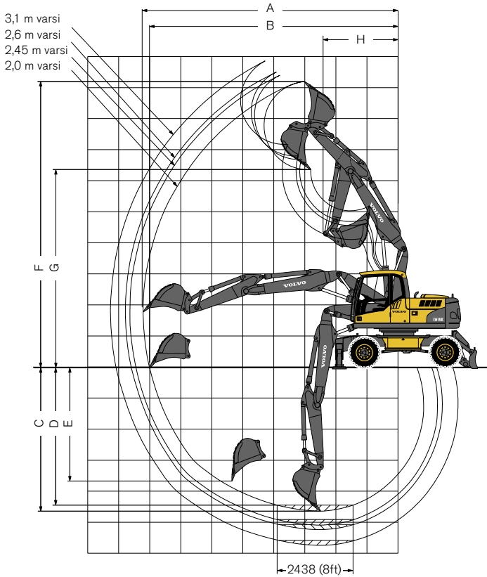
Kaksiosainen puomi 4,7 m ja varsi 2,0 m, 2,45 m, 2,6 ja 3,1 m
