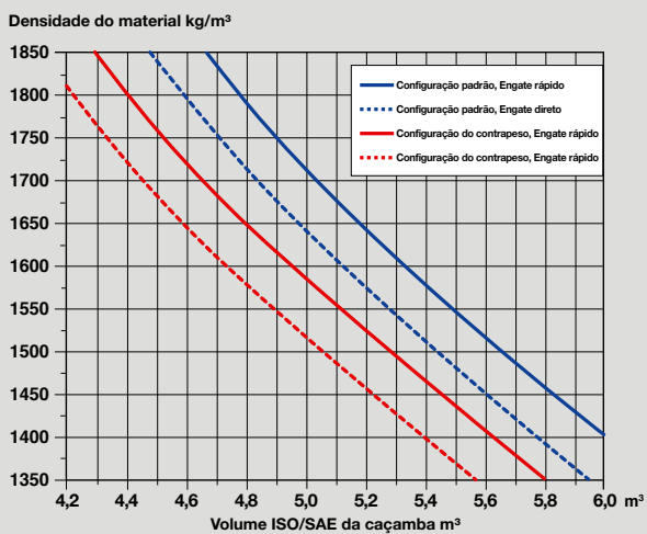
Caçamba para manuseio de agregados L180F, braço padrão, fator de enchimento 110%, pneus L3.
