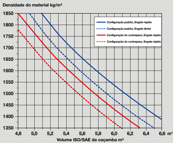
Caçamba para manuseio de agregados L220F, braço estándar, fator de enchimento 110%, pneus L4.
