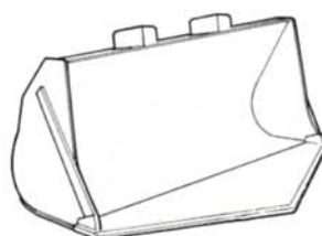
Spetsig skopa utan tänder. Lämplig för hårt material, grus och finsprängt berg, malm samt jordautäckning.
