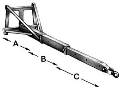
Kranarm, 3-delad, mek. Lyftkraft max räckvidd 850 kg
