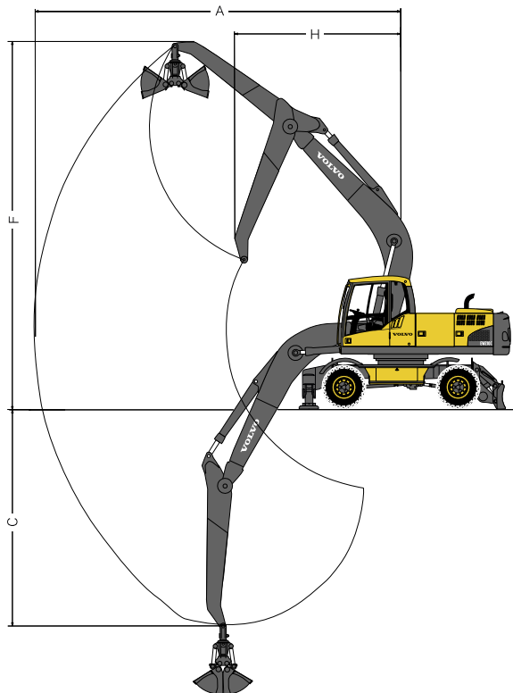
Flèche monobloc 5,6 m et balancier de 3,2 m pour pince
