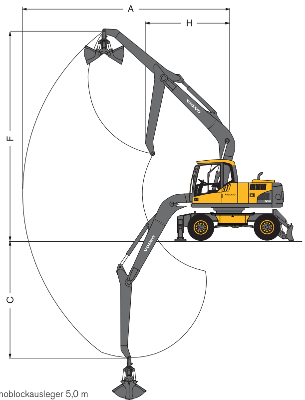
Monoblockausleger 5,0 m und Greiferstiel 2,95 m
