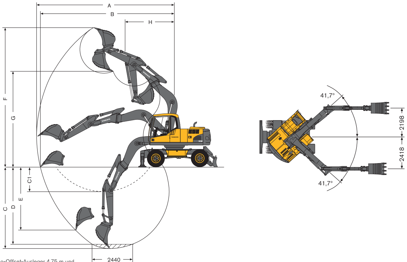
Mono-Offset-Ausleger 4,75 m und Stiel 2,0 m, 2,45 m, 2,6 m, 3,1 m
