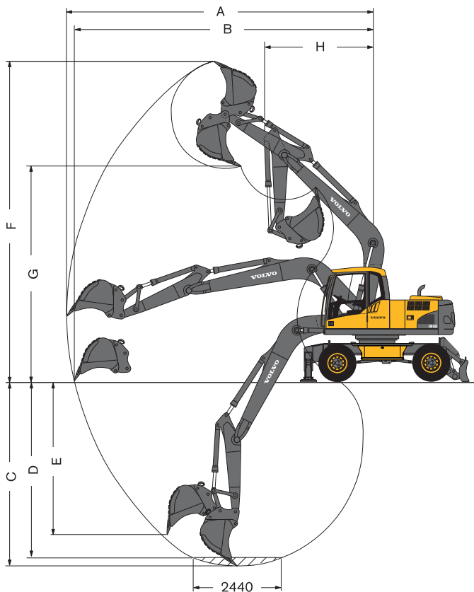
Monoblockausleger 5,0 m und Stiel 2,0 m, 2,45 m, 2,6 m, 3,1 m
