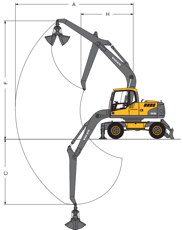
Pluma monobloque de 4,5 m y brazo de bivalva de 2,95 m
