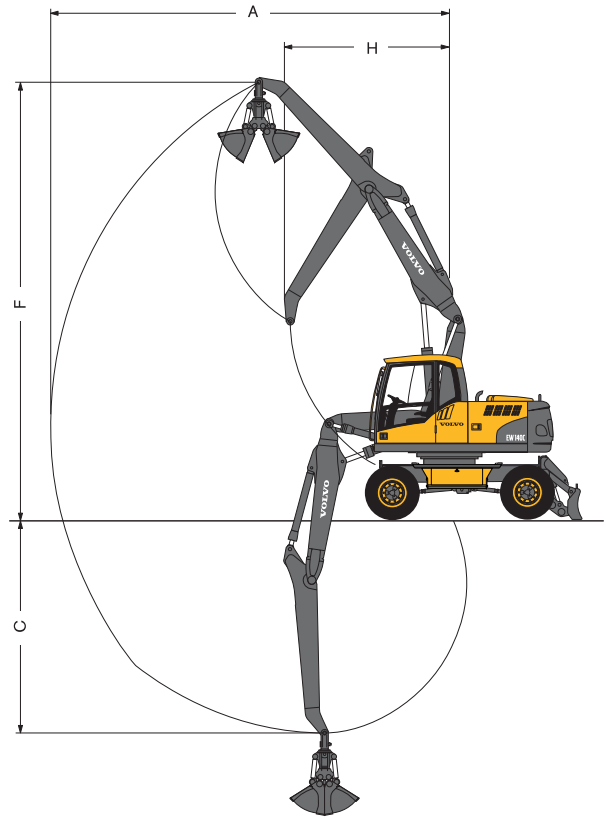
Pluma articulada de 4,7 m y brazo de bivalva de 2,95 m
