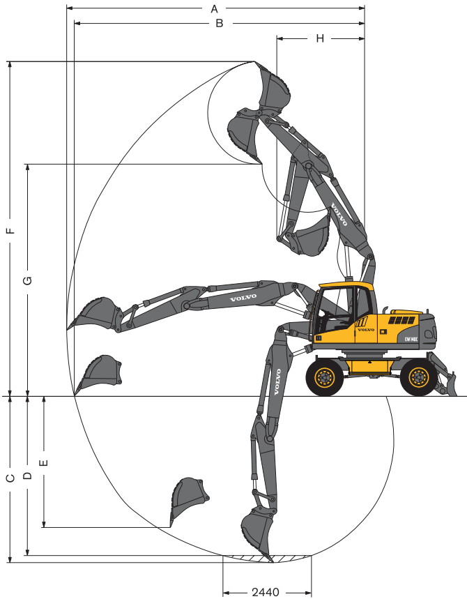
Pluma articulada de 4,7 m y brazo de 2,0 m, 2,45 m, 2,6 m, 3,1 m,
