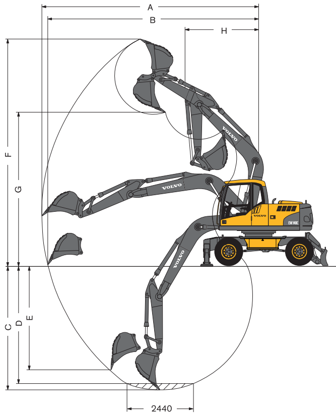
Pluma monobloque de 4,5 m y brazo de 2,0 m, 2,45 m, 2,6 m, 3,1 m
